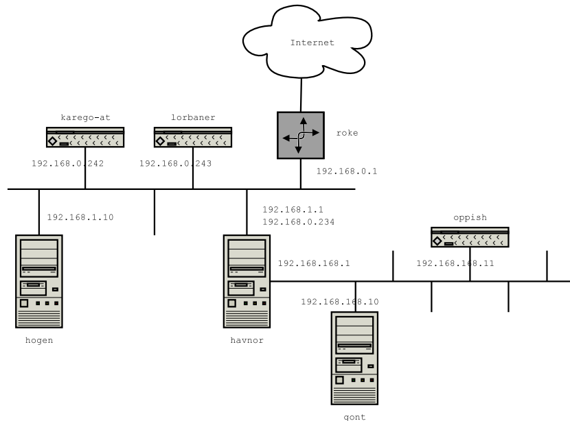
Figura 7.4: Schema di una rete di prova.
