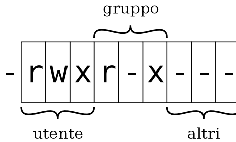
Figura 1.4: Legenda dei permessi dell'output di ls .
