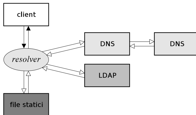
Figura 7.5: Schema di funzionamento delle funzioni del resolver .
