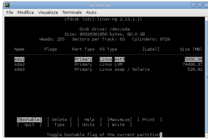
Figura 5.1: Schermata del comando cfdisk .
