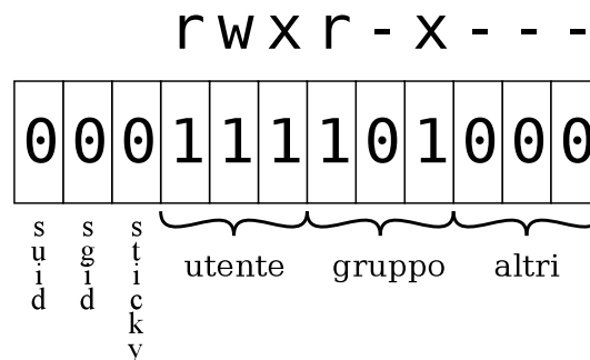
Figura 1.5: Schema dei bit dei permessi mantenuti nell' inode .
